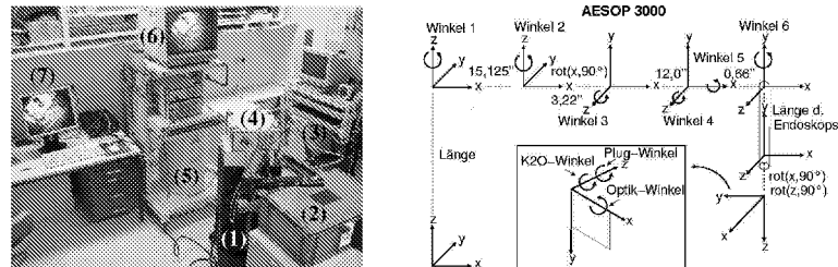
Abb. 1. Laboraufbau (links) und Kinematik des Roboterarms AESOP 3000 (rechts). Links: (1) AESOP 3000 (2) „Patient“ (3) Kamerakopf und Endoskop (4) Lichtquelle (5) Computer (6) Endoskopieturn mit Monitor (Originalbild) (7) Zweiter Monitor (Computerbild/Lichtfeld). Rechts: Sieben Freiheitsgrade (Länge, Winkel 1, . . . , 6), Länge d. Endoskops, Korrekturwinkel (K2O-, Plug- und Optik-Winkel)
